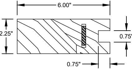
⑱ ASTRAGAL WOOD (0.44 MIN. S.G.)
