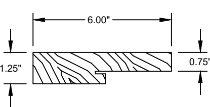
⑲ DOOR FRAME JAMB WOOD
