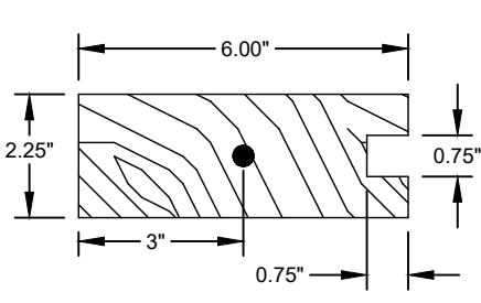
④ TOP RAIL - OPAQUE DOOR WOOD (0.44 MIN. S.G.)
